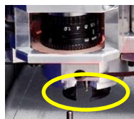
Frästiefenbegrenzer für Protomat S depth limiter (Protomat S)
